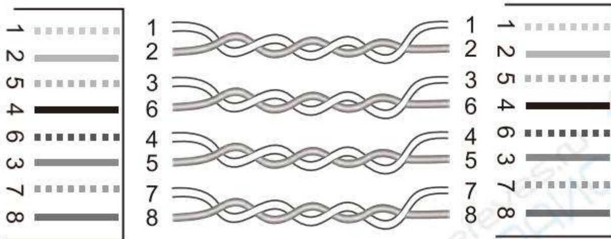
Схема подключения раздельной пары
