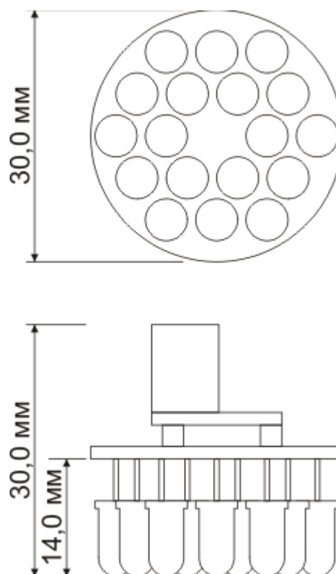
Габаритные размеры
