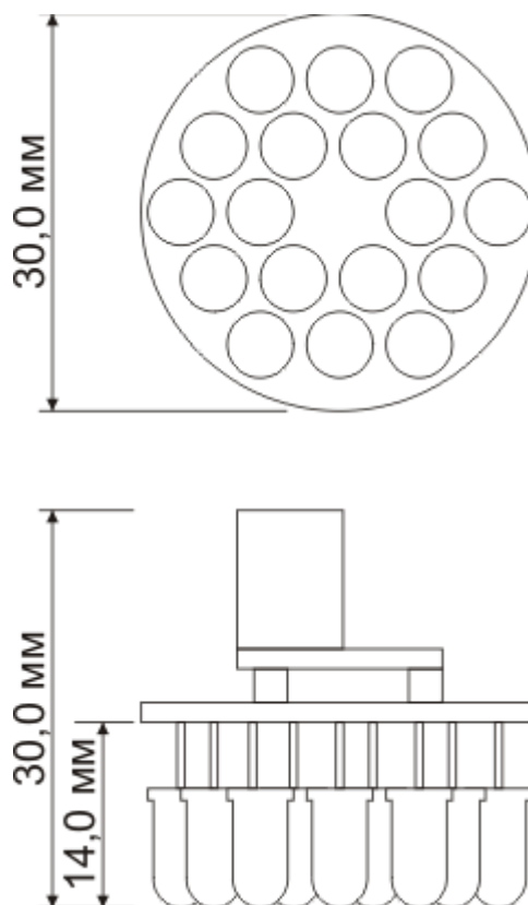
Габаритные размеры
