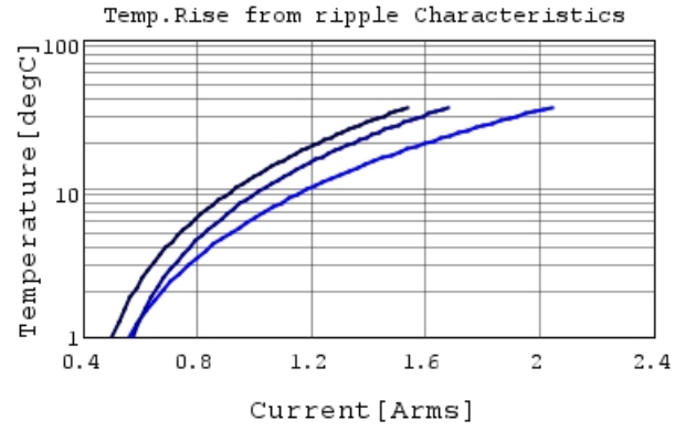
GQM1875C2E560GB12 Temp.rise — 300MHz —
