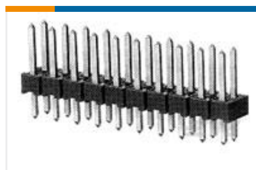
TE Part #826632-1 1P AMPMODU II PIN HDR
