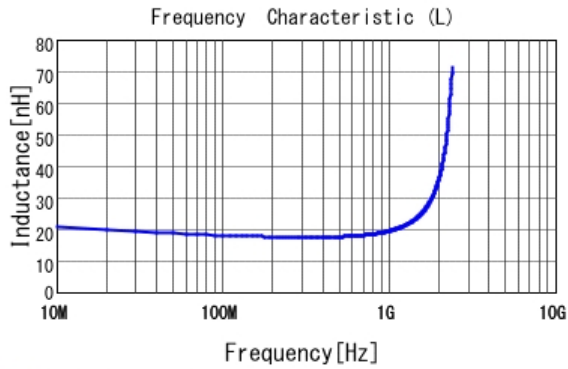
■ LQG15HN18NH02 L
