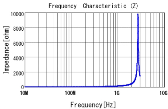
■ LQG15HN18NH02 |Z|
