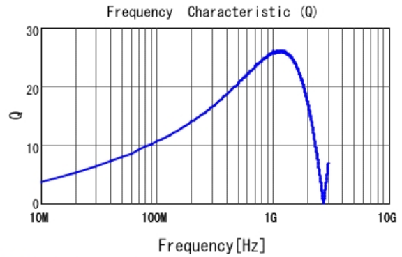
■ LQG15HN18NH02 Q
