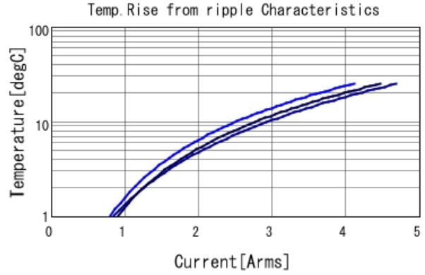
KCM55WR71J226MH01 Temp. rise ■ 50kHz ■ 100kHz ■ 300kHz
