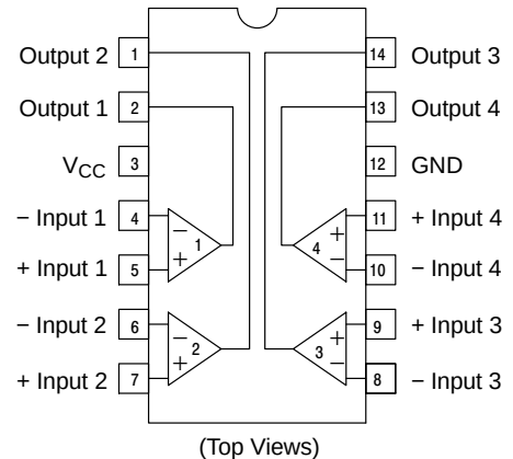
SOIC-14 / TSSOP-14
