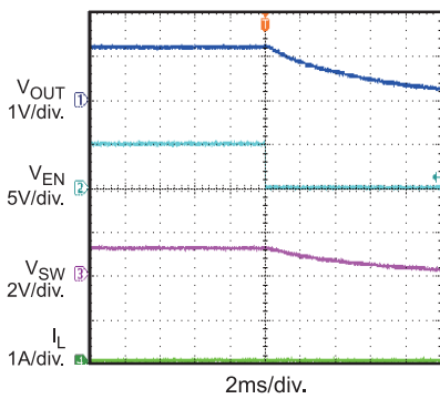
Enable Shutdown I_{OUT} = 0A , PFM
