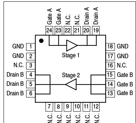
QFN 4 × 4
