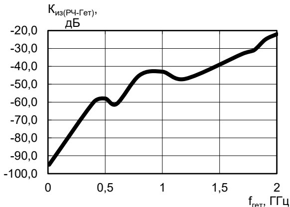
Зависимость коэффициента изоляции входа РЧ от гетеродина от частоты сигнала гетеродина ( U_n = 5 \text{ В} , f_{ПЧ} = 10 \text{ МГц} , P_{РЧ} = -20 \text{ дБм} , P_{ГЕТ} = 0 \text{ дБм} )
