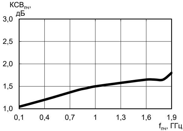
Зависимость КСВ ПЧ от частоты сигнала ПЧ ( U_n = 5 \text{ В} , f_{\text{ПЧ}} = 10 \text{ МГц} , P_{\text{ГЕТ}} = 0 \text{ дБм} )
