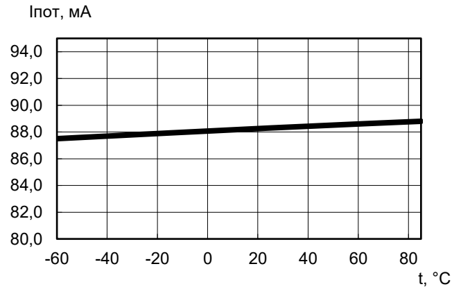
Зависимость тока потребления от температуры ( U_n = 5 \text{ В} )
