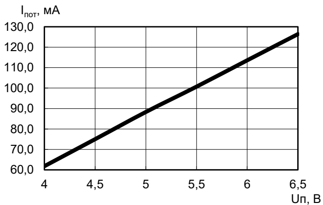
Зависимость тока потребления от напряжения питания ( T = +25 \text{ °C} )
