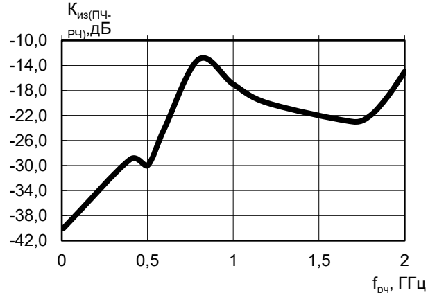
Зависимость коэффициента изоляции выхода ПЧ от РЧ от частоты сигнала РЧ ( U_n = 5 \text{ В} , f_{ПЧ} = 10 \text{ МГц} , P_{РЧ} = -20 \text{ дБм} , P_{ГЕТ} = 0 \text{ дБм} )
