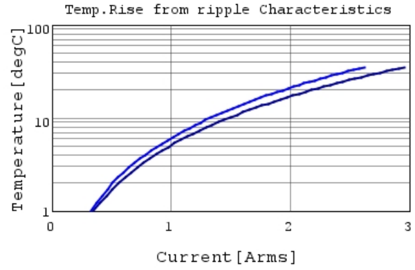
GCM188R71E105KA64 Temp.rise — 500kHz
