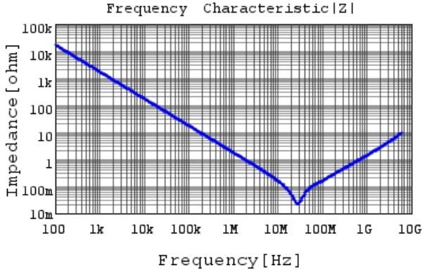
GCM155R71H104KE02 |Z| DC0V, 25degC
