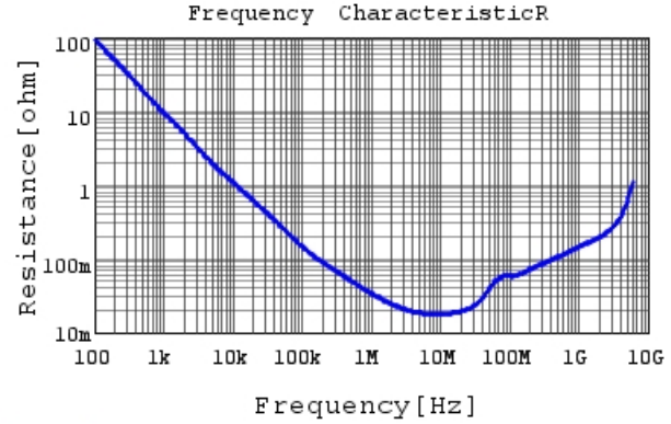
GCM155R71H104KE02 R DC0V, 25degC
