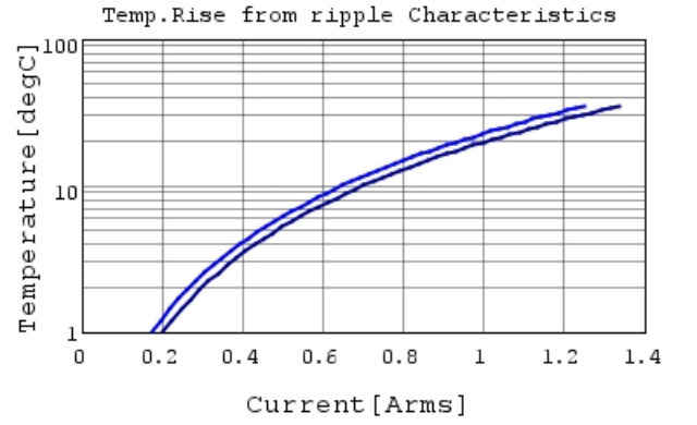
GCM155R71H104KE02 Temp.rise — 800kHz —
