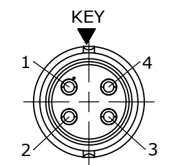
WIRING END W6282-4SG-P-5XX
