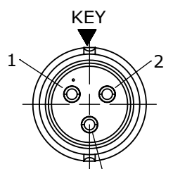
WIRING END W6282-3SG-P-5XX
