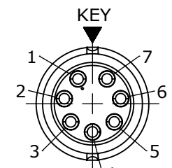
WIRING END W6282-7SG-P-5XX
