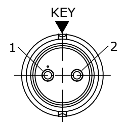
WIRING END W6282-2SG-P-5XX
