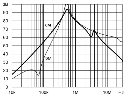
FN 3287: 63 A
