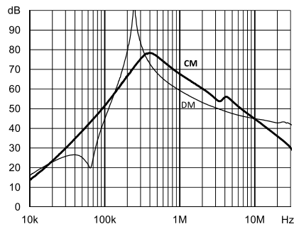
FN 3287: 160 A
