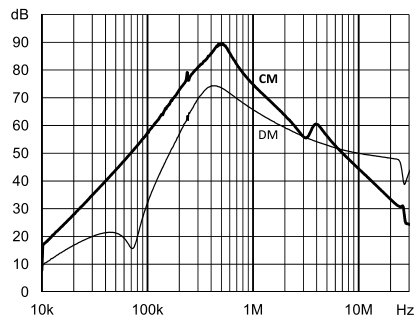
FN 3287: 80 A
