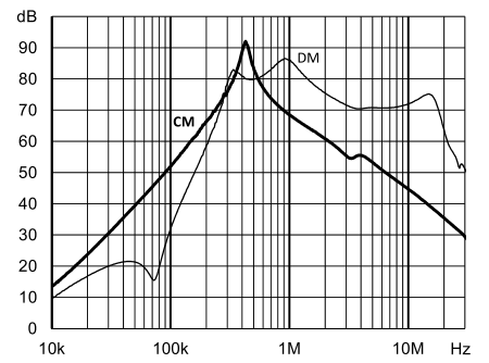
FN 3287: 100 A
