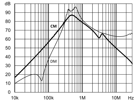
FN 3287: 50 A
