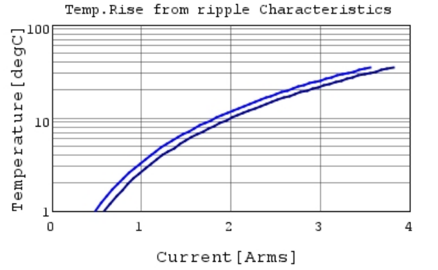
GRM188R61E225MA12 Temp.rise 500kHz
