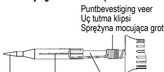
Soldeerpunt Hava Ucu Grot lutownicy Klemgroef Sıkıştırma vidası Szczelina zaciskowa Puntbevestiging veer Uç tutma klipsi Sprężyna mocująca grot Verwarmingselement Isıtıcı gövde Grzejnik
