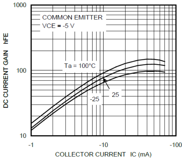
Fig. 10.15 RN2318 h_{FE}-I_c
