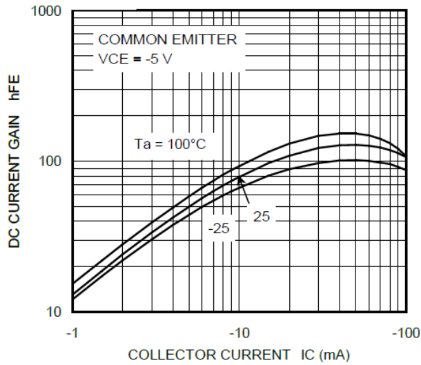
Fig. 10.13 RN2316 h_{FE}-I_c
