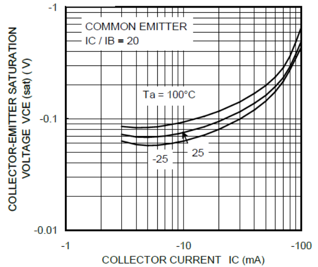
Fig. 10.18 RN2316 V_{CE(sat)}-I_c
