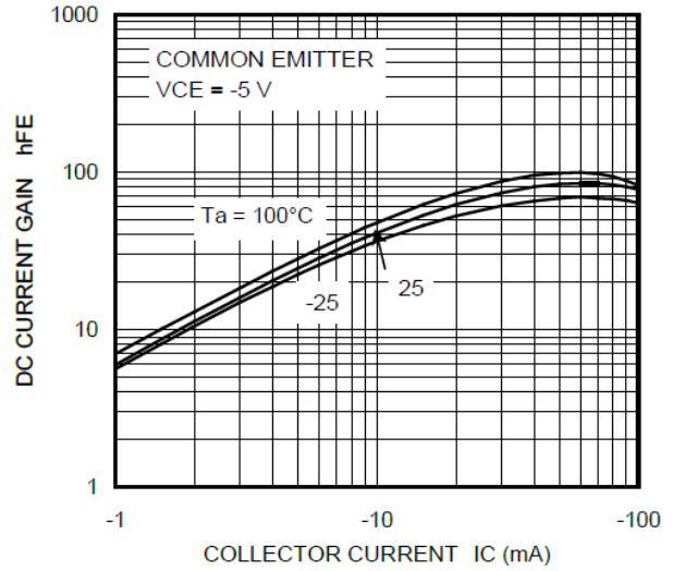
Fig. 10.14 RN2317 h_{FE}-I_c
