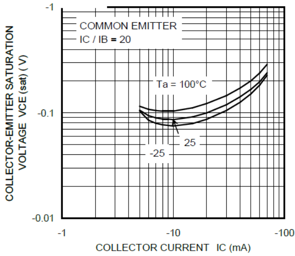
Fig. 10.19 RN2317 V_{CE(sat)}-I_C
