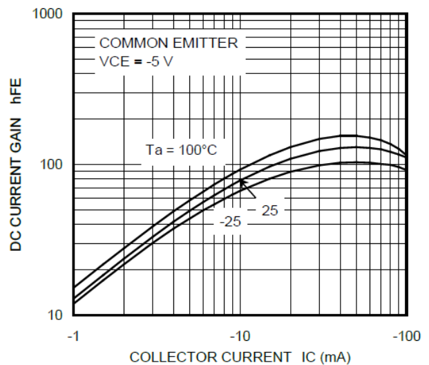
Fig. 10.12 RN2315 h_{FE} - I_C
