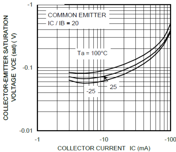
Fig. 10.17 RN2315 V_{CE(sat)}-I_c
