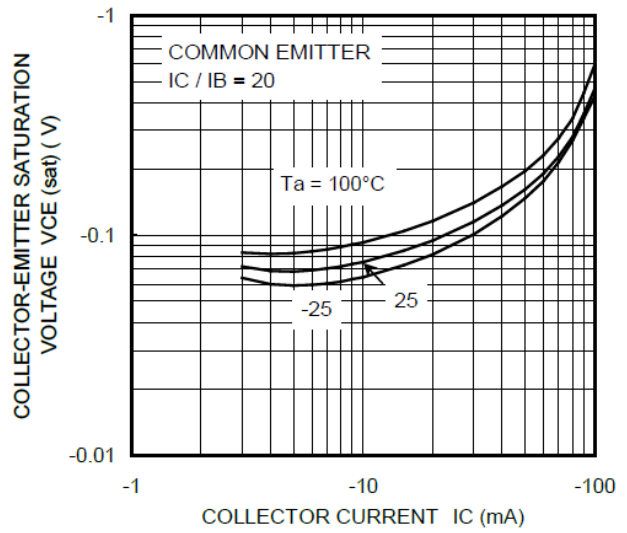
Fig. 10.16 RN2314 V_{CE(sat)}-I_c
