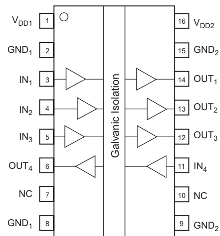
HCPL-902J/-092J
