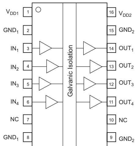
HCPL-900J/-090J
