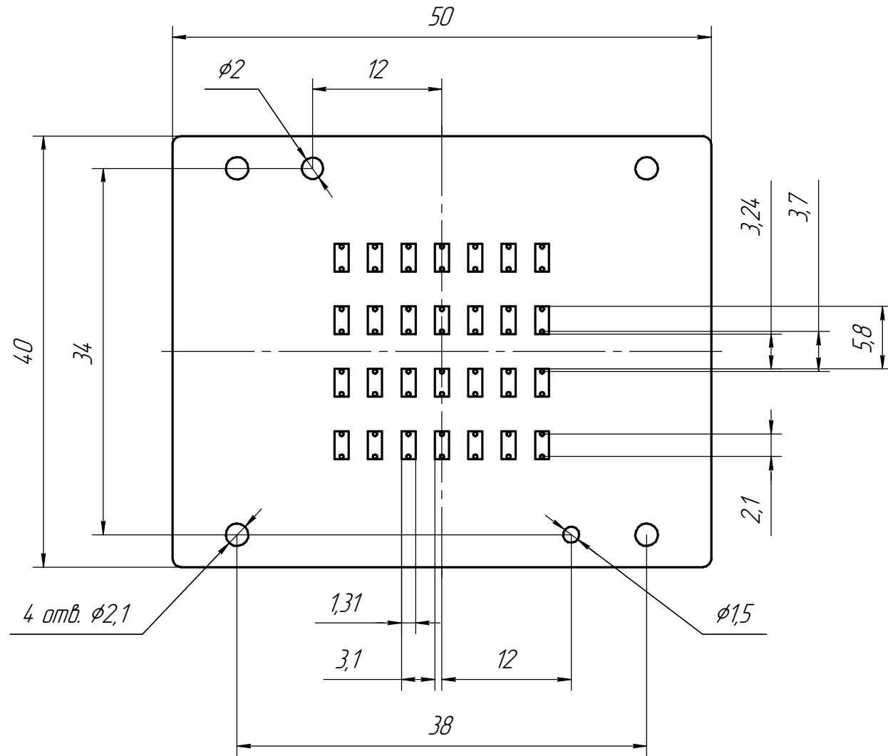
Посадочное место, вид сверху (2:1)
