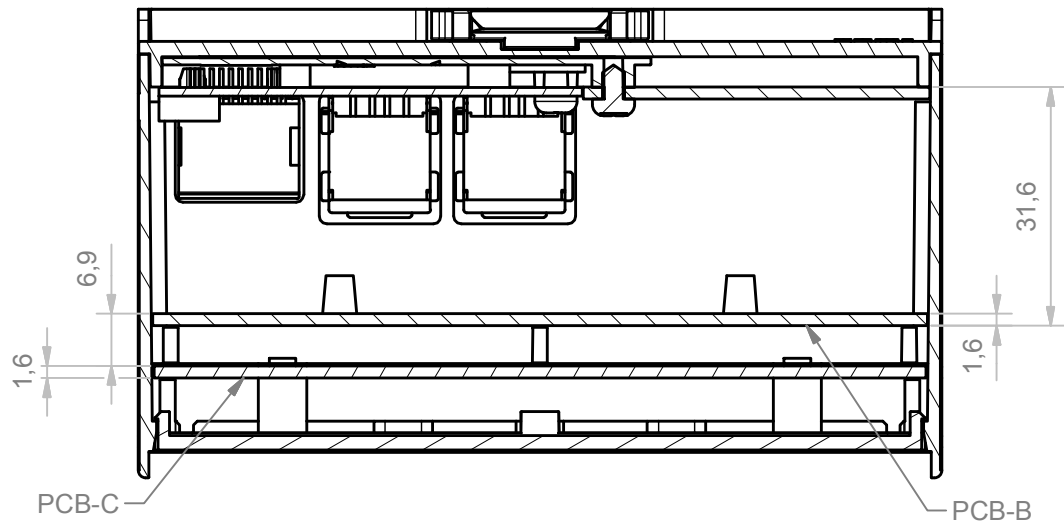
A-A (1:1)
