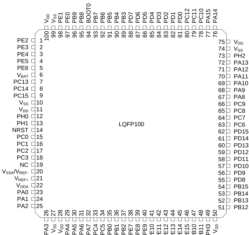
图 3. AT32F435/437 系列 LQFP100 引脚分布
