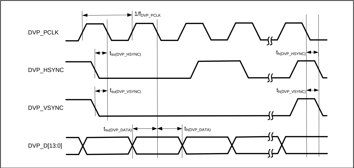
图 52. DVP 时序图
