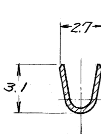
断面 B-B
