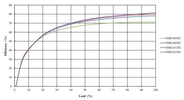
24V Inputs
