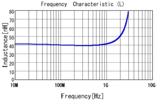
■ LQW15AN40NJ00 L
