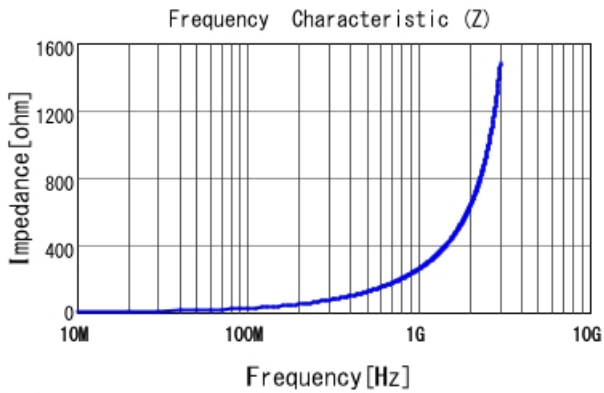
■ LQW15AN40NJ00 |Z|
