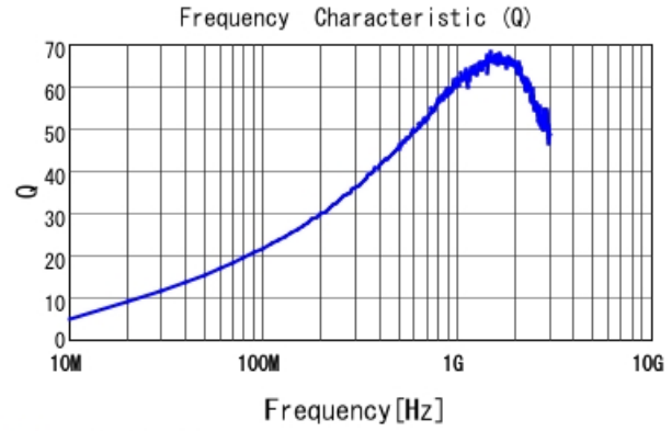
■ LQW15AN40NJ00 Q
