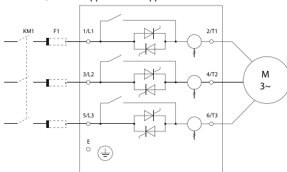
Рисунок 2 – Подключение силовых клемм
