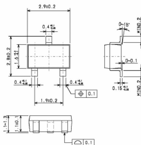
SOT23-3/SOT23-3B
