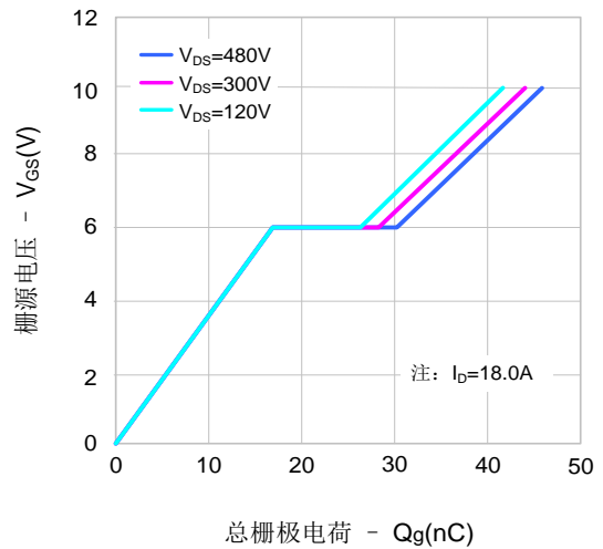
图6. 电荷量特性
