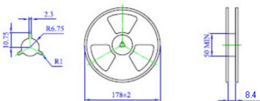
Reel dimensions
