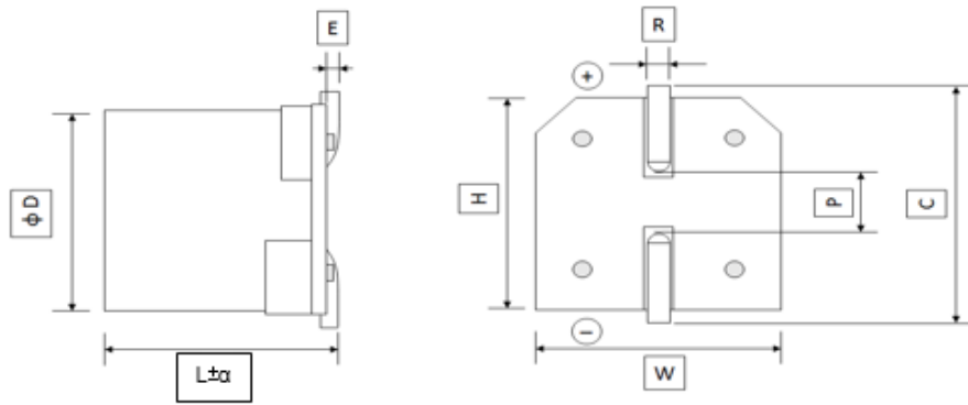
Fig. 2 Dimension
