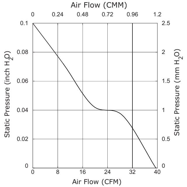
CFM-9225V-130-340
