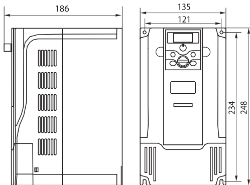
Габарит корпуса 4
