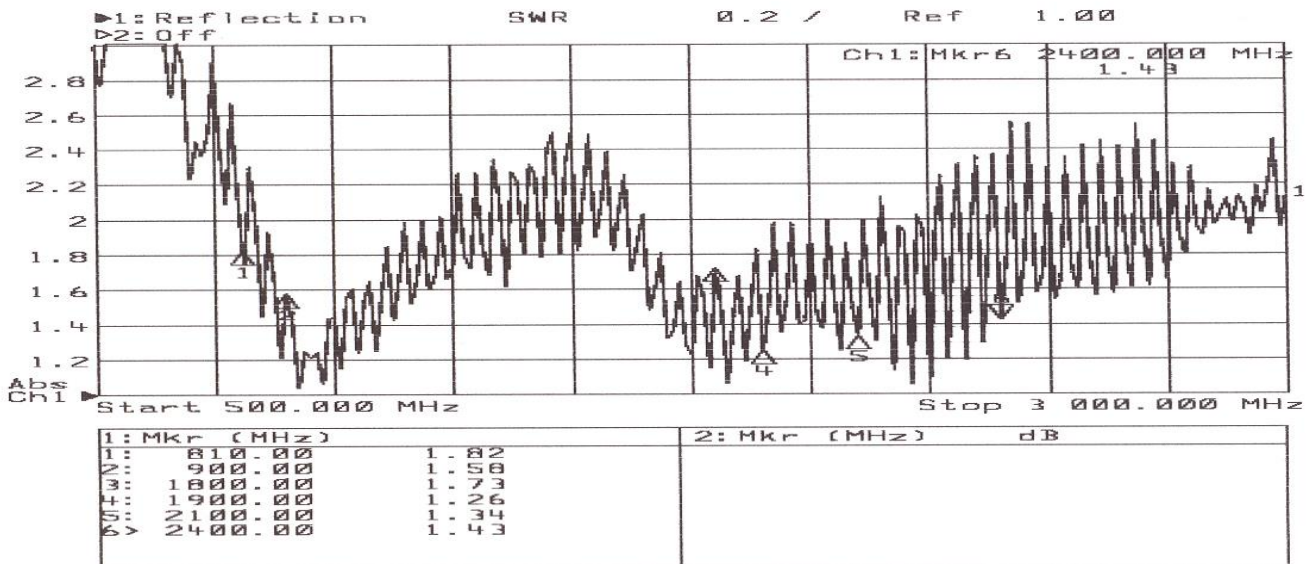
Figure 1 VSWR 500MHz – 3000MHz
