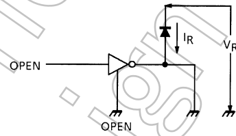
6. I_R
