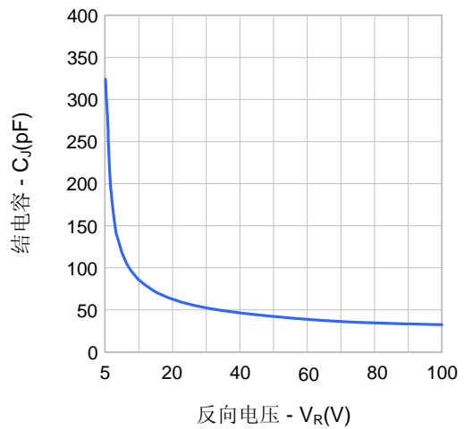
图 4: 结电容特性
