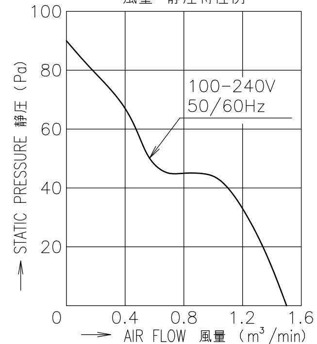
風量-静圧特性例
