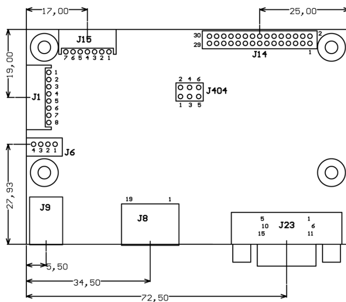
Рисунок 4 - Габаритный чертёж контроллера NT11H
