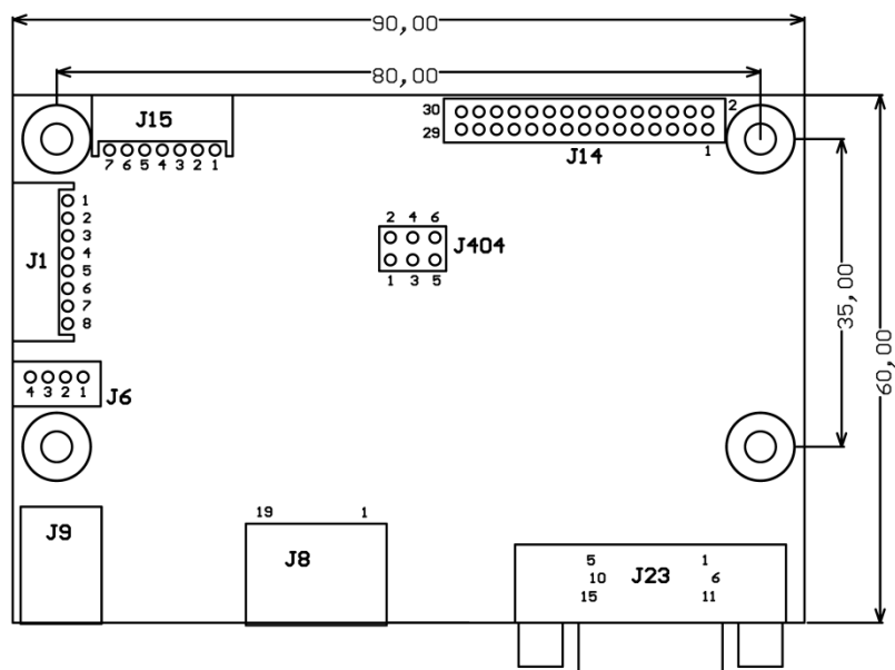
Рисунок 4 - Габаритный чертёж контроллера NT11H
