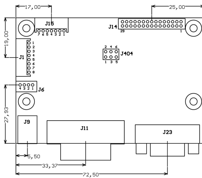
Рисунок 2 - Габаритный чертёж контроллера NT11S
