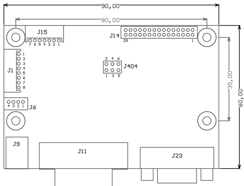
Рисунок 2 - Габаритный чертёж контроллера NT11S
