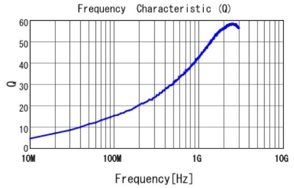
■ LQG15HN2N7S02 Q
