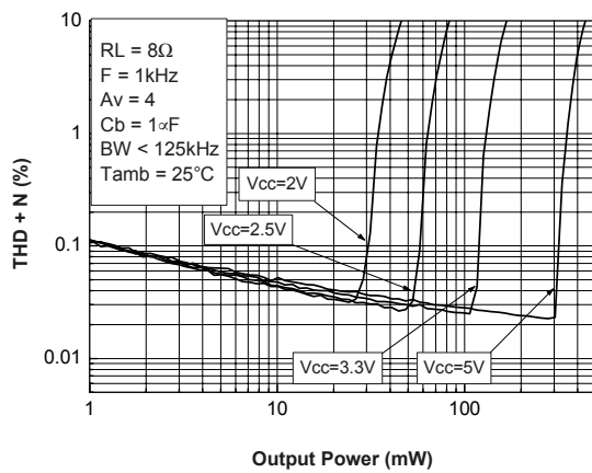
Figure 59. THD + N vs. output power RL = 8 Ω, Av = 4
