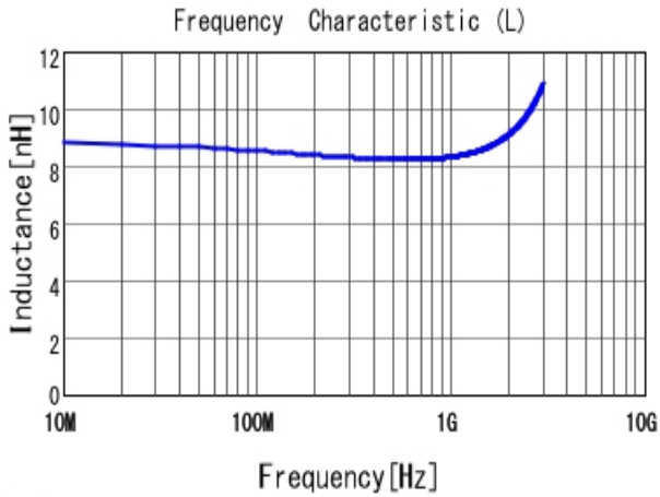
■ LQP03TN8N2H02 L
