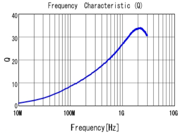
■ LQP03TN8N2H02 Q
