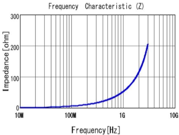
■ LQP03TN8N2H02 |Z|
