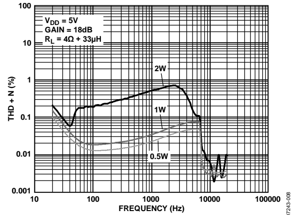
Figure 8. THD + N vs. Frequency, VDD = 5 V, RL = 4 Ω + 33 μH, Av = 18 dB
