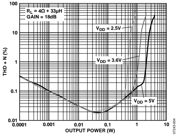
Figure 4. THD + N vs. Output Power into 4 Ω + 33 μH, Av = 18 dB
