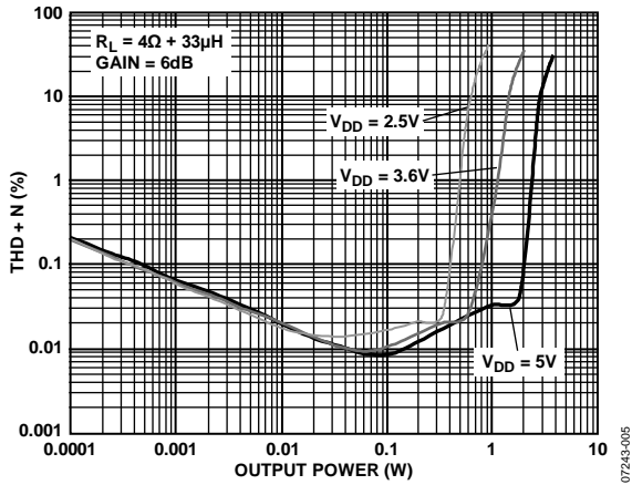
Figure 5. THD + N vs. Output Power into 4 Ω + 33 μH, Av = 6 dB
