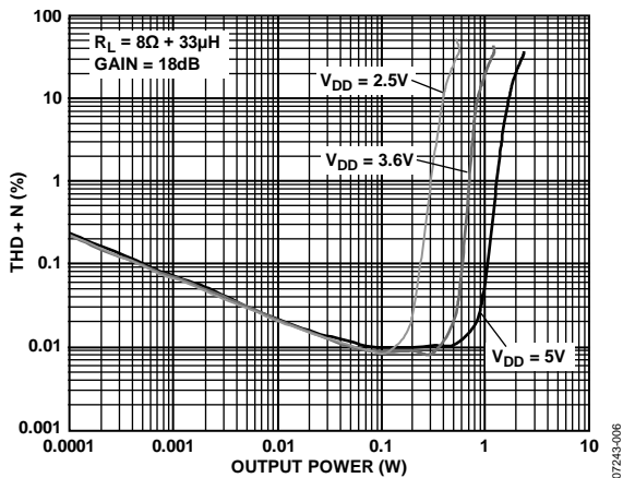
Figure 6. THD + N vs. Output Power into 8 Ω + 33 μH, Av = 18 dB
