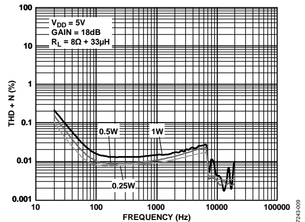
Figure 9. THD + N vs. Frequency, VDD = 5 V, RL = 8 Ω + 33 μH, Av = 18 dB
