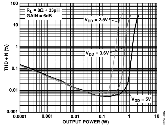
Figure 7. THD + N vs. Output Power into 8 Ω + 33 μH, Av = 6 dB
