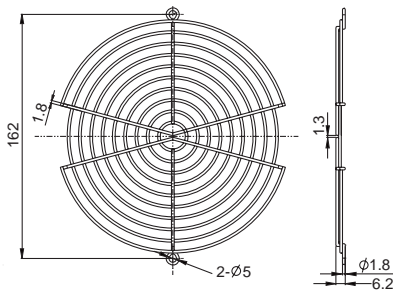
FG-17B For 172mm Fan
