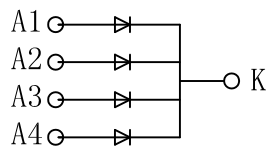
背光电路图
