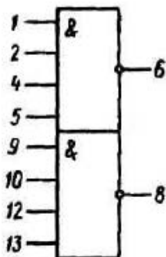
Условное графическое обозначение К555ЛА7
