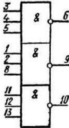
Условное графическое обозначение КР1561ЛА9, КФ1561ЛА9
