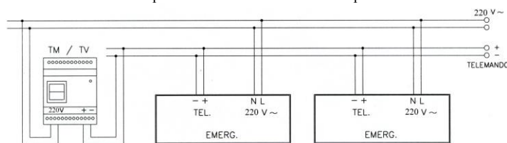
Рис. II - Схема подключения светильников с люминесцентными лампами непостоянного действия.
