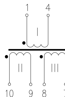
Схема электрическая
