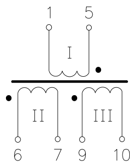
Схема электрическая
