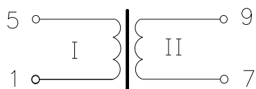
Схема электрическая
