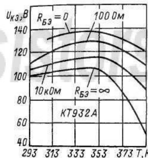
Зависимость напряжения коллектор-эмиттер от температуры.
